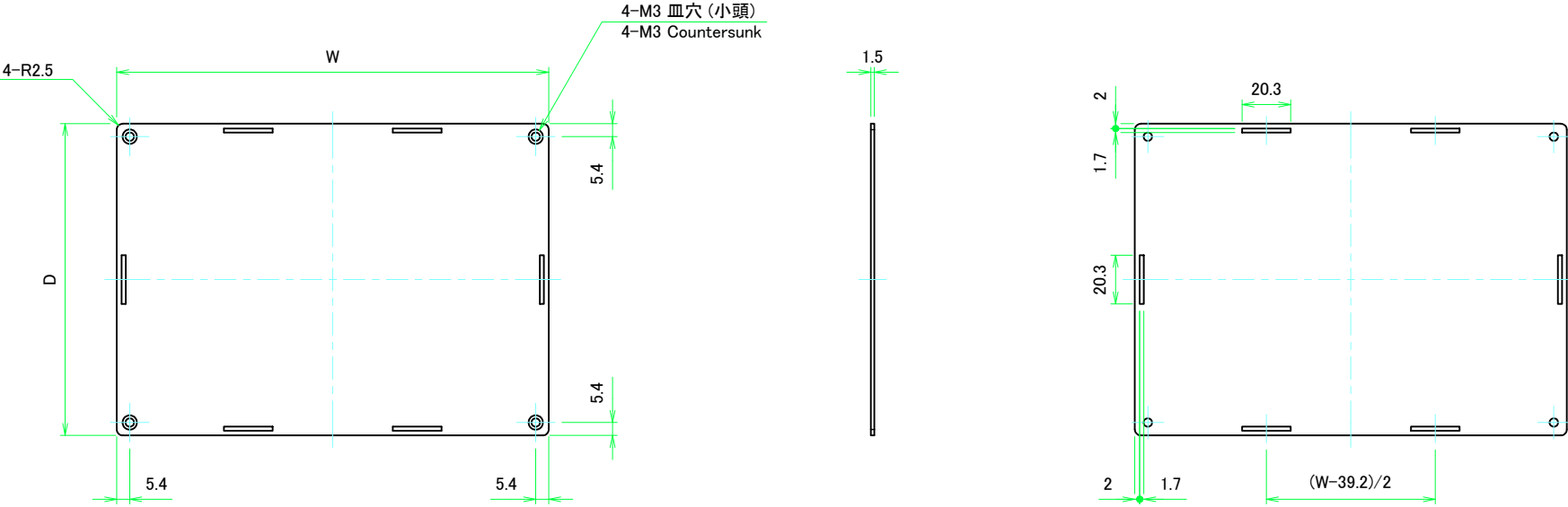
上カバー裏面 / Top cover Backside
