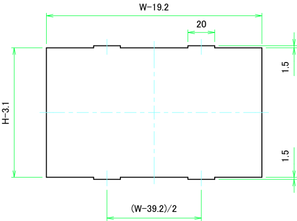
Wパネル1表面 / W Panel 1 Frontside
